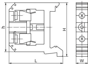
Рис. 1 Габаритные размеры
