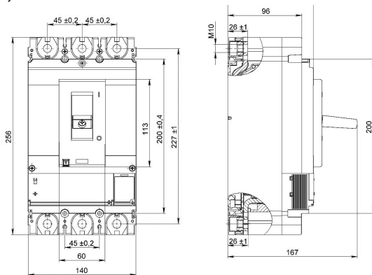
Рисунок 4 – Габаритные, установочные и присоединительные размеры выключателей
