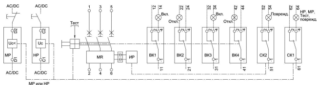
а) с микропроцессорными распределителями
