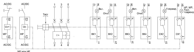
б) с термомангнитными распределителями
