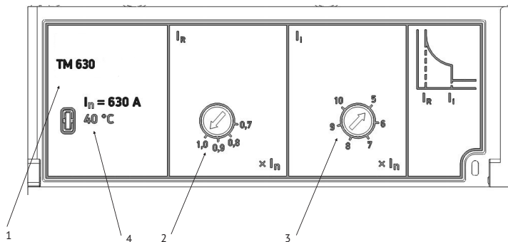
Рисунок 1 – Общий вид лицевой панели термомагнитных расцепителей тока
