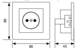
РОЗЕТКА ОДНОМЕСТНАЯ Б/З
