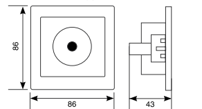
РОЗЕТКА ТЕЛЕВИЗИОННАЯ, КОМПЬЮТЕРНАЯ, КОМПЬЮТЕРНАЯ ДВОЙНАЯ
