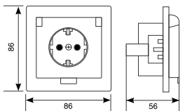
РОЗЕТКА ОДНОМЕСТНАЯ С ПРОЗРАЧНОЙ КРЫШКОЙ С/З
