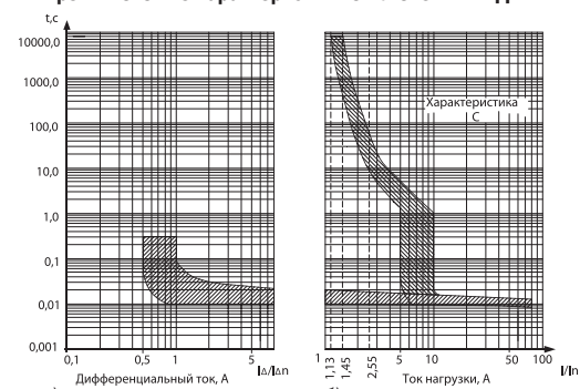
а) Характеристика отключения и пределы времени срабатывания по дифференциальному току.
