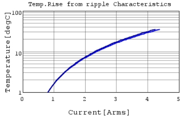
GRM188C81E475KE11 Temp.rise — 500kHz
