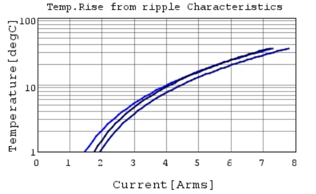
GRM32EE70G107ME19 Temp.rise 50kHz
