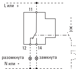
Рис. 1 Схема подключения
